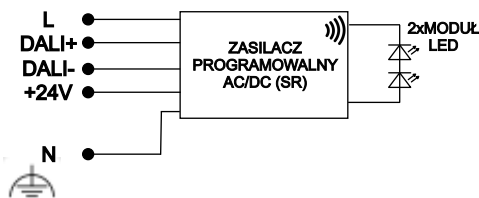
1. Źródło światła LED (I Klasa ochronności) (wersja podstawowa - zasilacz programowalny)
